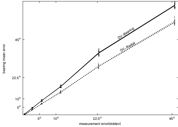
Fig. 13 HEADING ERROR
