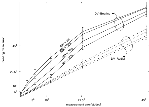
Fig. 13 HEADING ERROR
